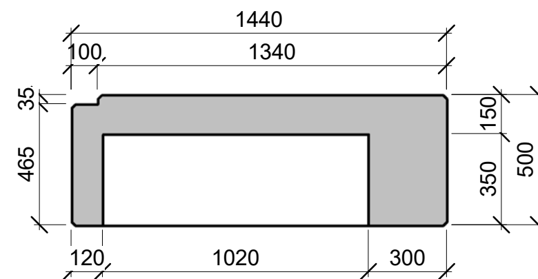
2 Section 1 1 : 20
